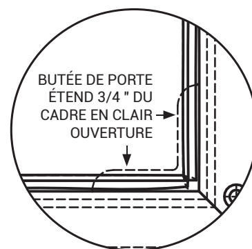
DETALLE DEL TOPE DE PUERTA
