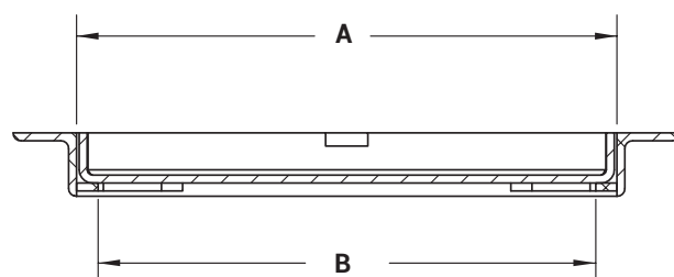
SECCIÓN A-A
