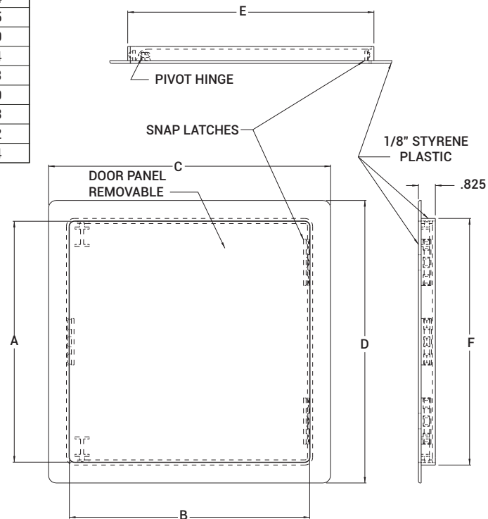
PA-3000 Vista de parte trasera de la puerta
