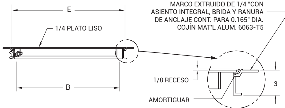
DETALLE DEL MARCO
