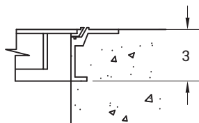
DETALLE DEL MARCO
